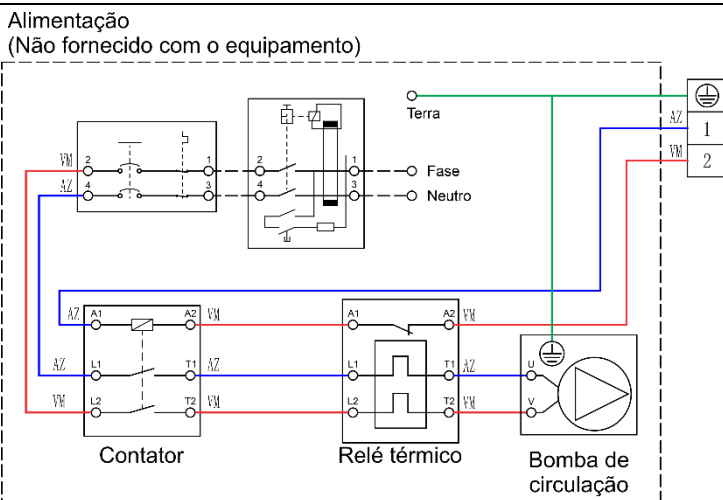
Figura 11 – Instalação elétrica da bomba de circulação
