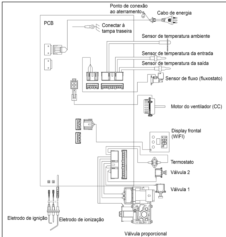
Fig. 3 Esquema funcional 21 e 26L
