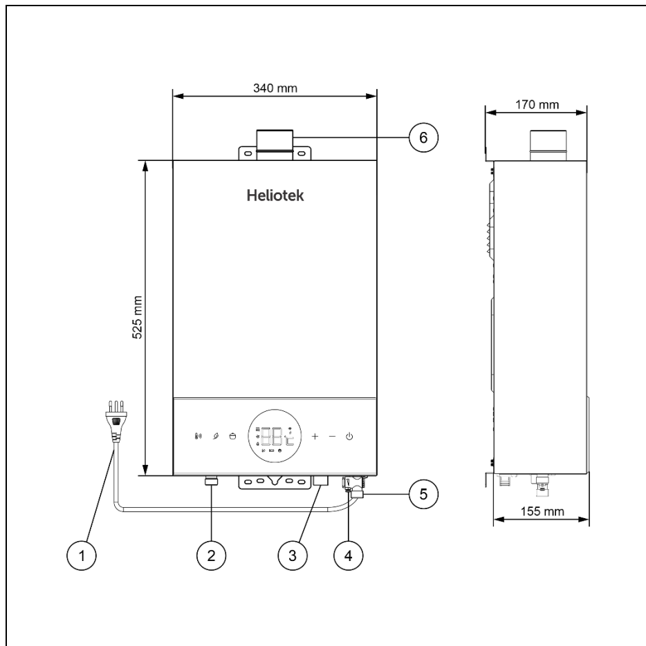
Fig. 1 Dimensões 21 e 26L
