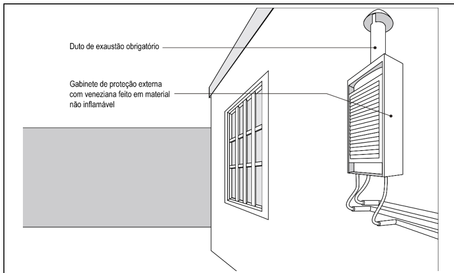
Fig. 7 Instalação em área externa
