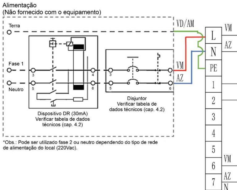
Figura 12 – Instalação elétrica da bomba de calor
