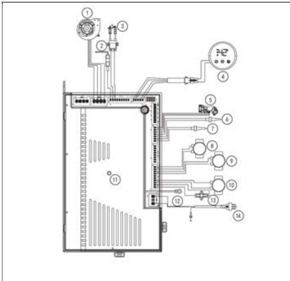
Fig. 6 Esquema funcional GWE-16 e GWE-21
