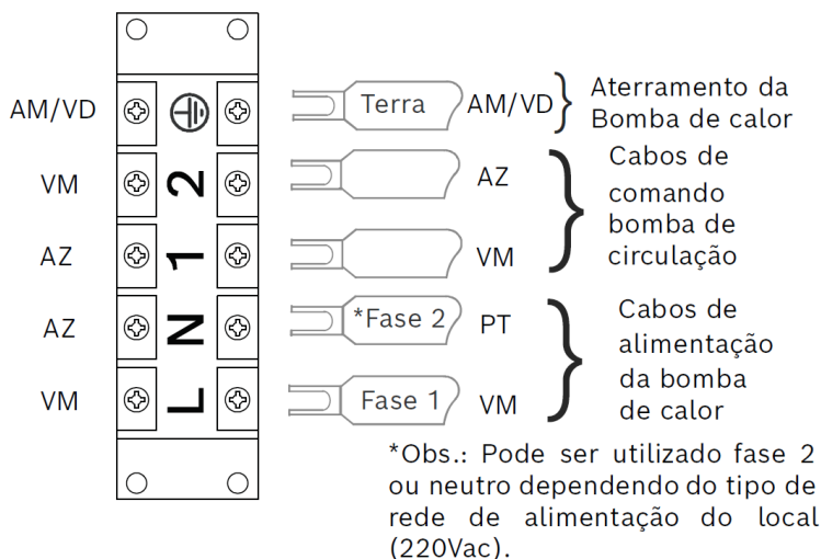
Figura 13 – Instalação dos cabos elétricos da bomba de calor
