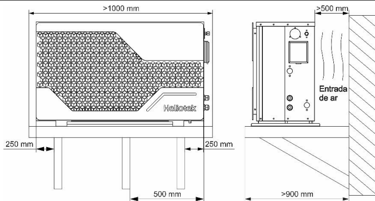
Figura 4 – Distâncias mínimas para instalação em parede ou áreas suspensas
