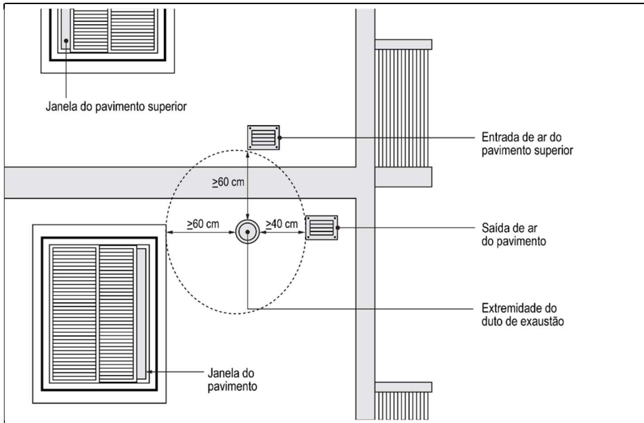
Fig. 16 Instalação típica de terminal
