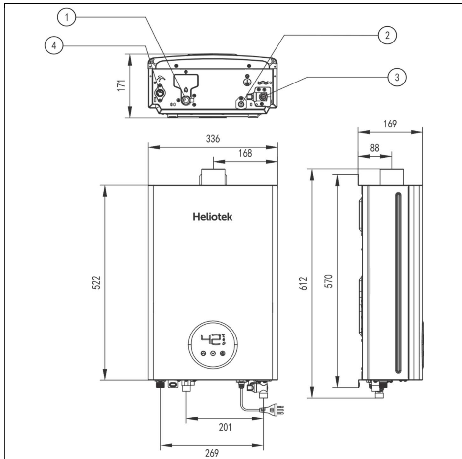
Fig. 1 Dimensões GWE-16
