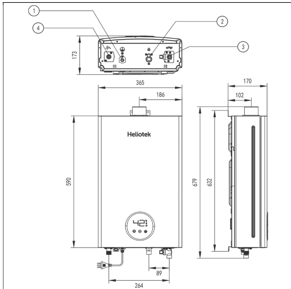
Fig. 2 Dimensões GWE-21
